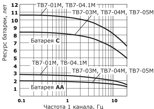
Рис. 1.1 – Ресурс батареи
