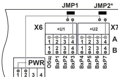
Рис. 4.5 – Организация питания датчиков давления
