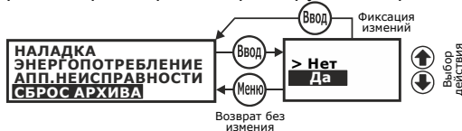
Рис. 3.4 – Сброс архива
